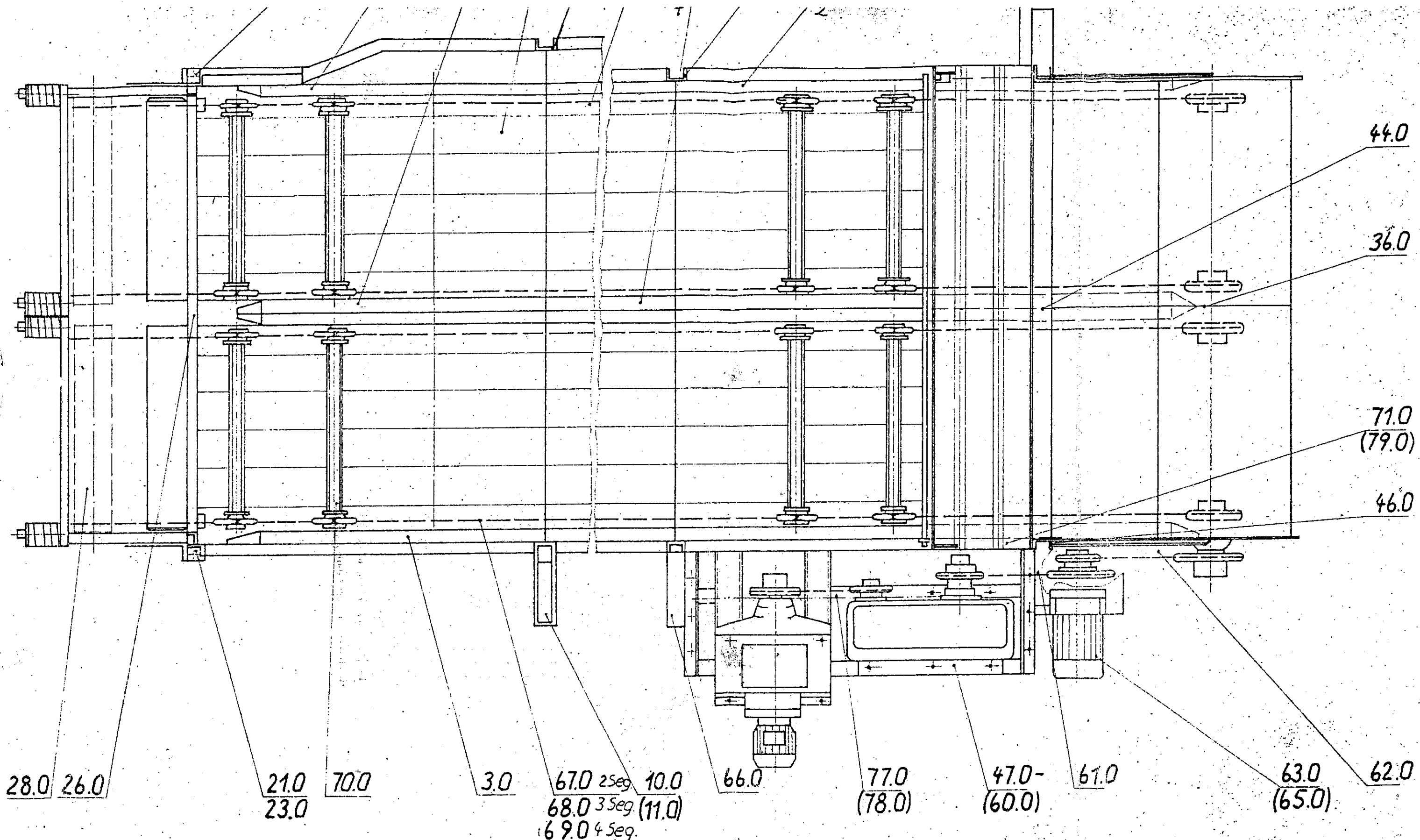
Grobfutterdosierer H110 Breit (2650 mm) (Ersatzteilzeichnung)
